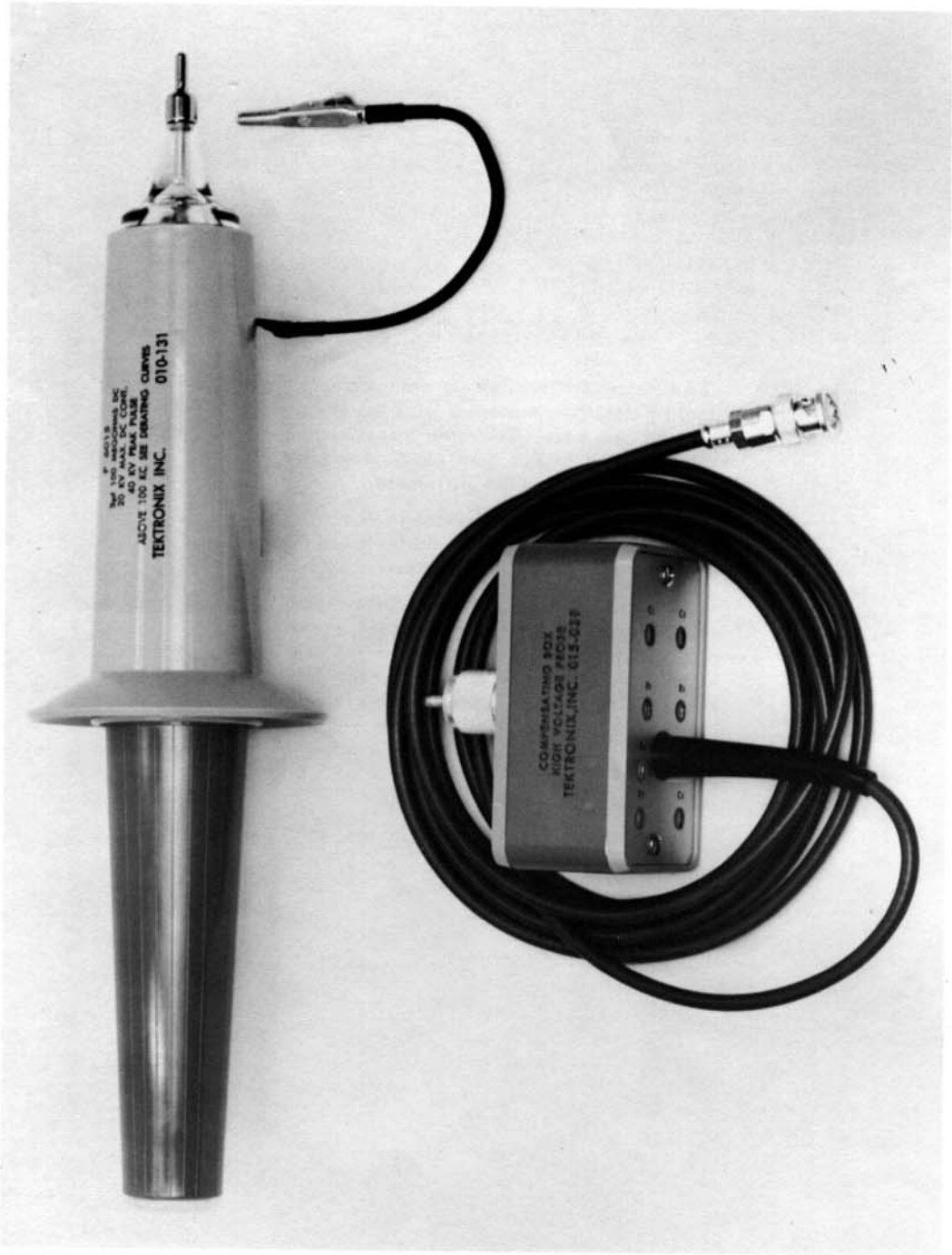
Fig. 1-1. P6015 Probe.
